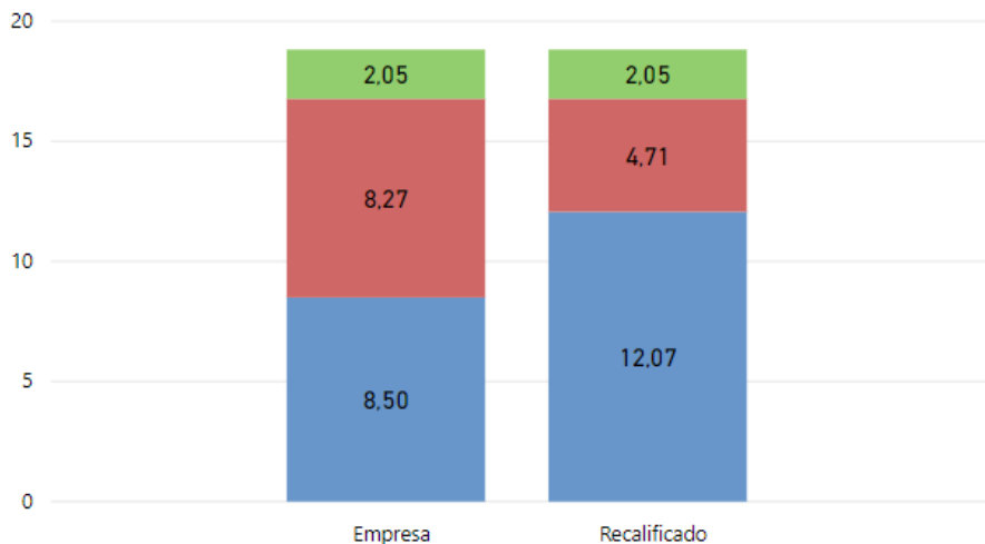
SAIDI Anual 2017
