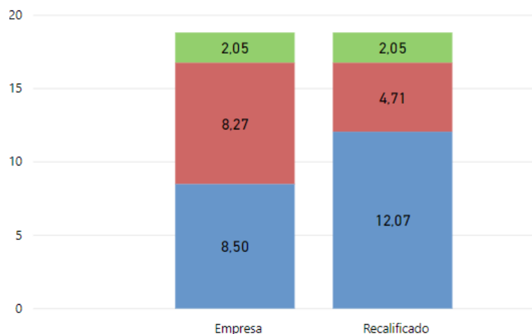
SAIDI Anual 2017
