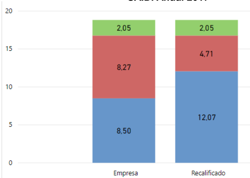
SAIDI Anual 2017
