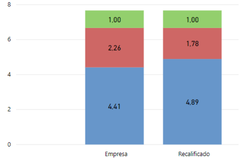
SAIDI 2018 ( Enero—Julio )
