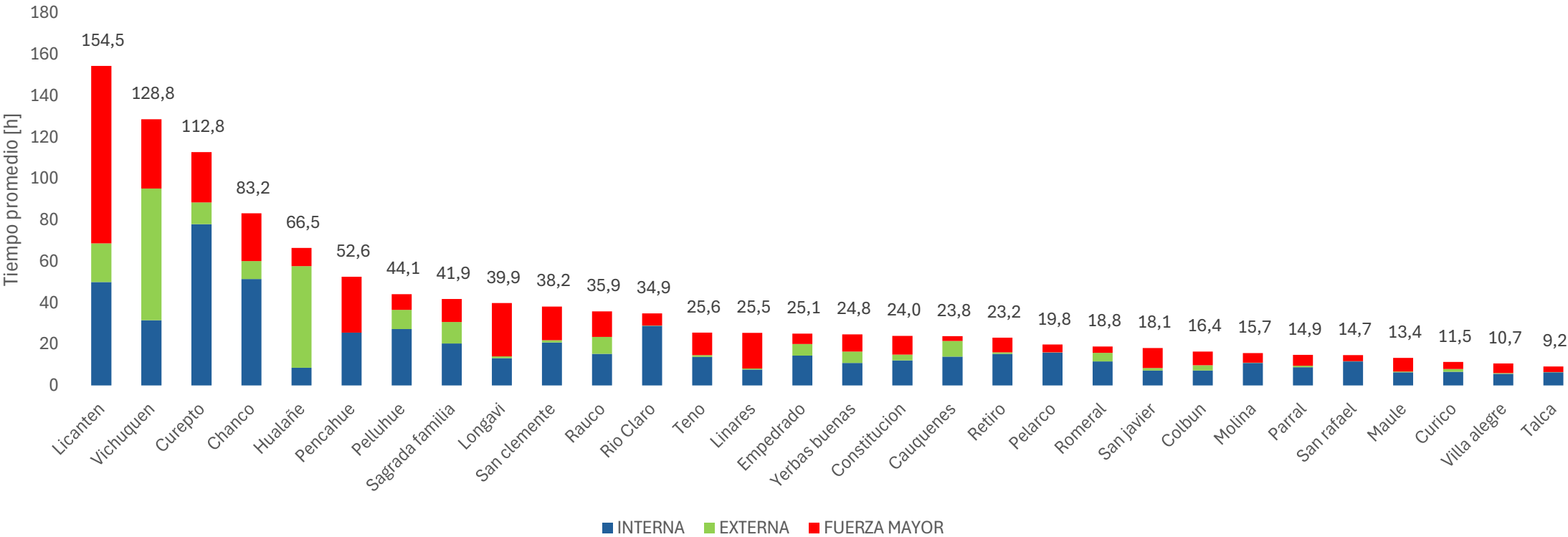
SAIDI por comuna región del Maule
