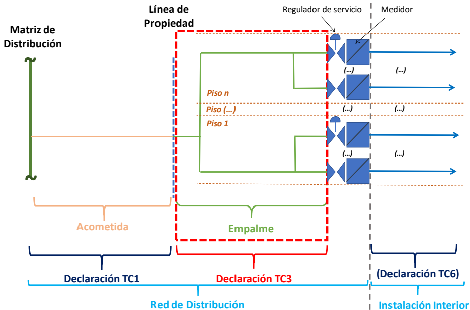
Figura 2: Alcance del trámite de declaración TC3 para el caso de un empalme múltiple.
