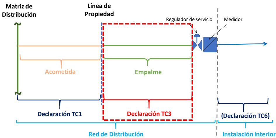
Figura 1: Alcance del trámite de declaración TC3 para el caso de un empalme individual.
