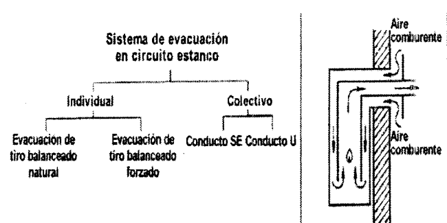
Figura 11. Sistemas de Evacuación - c) Circuito Estanco.
