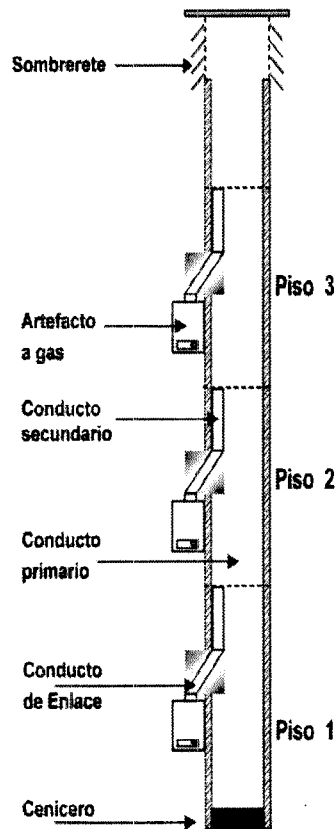
Figura 2. Conducto Colectivo de Evacuación de Gases Producto de la Combustión.
