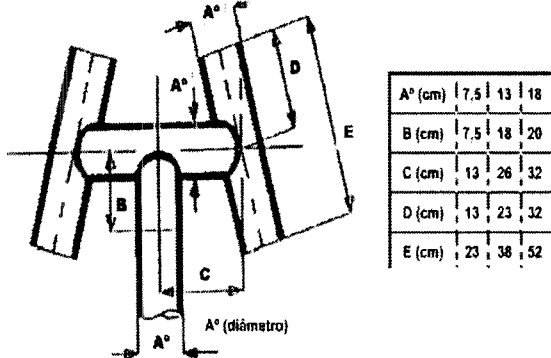
Figura 30. Sombrerete H.
