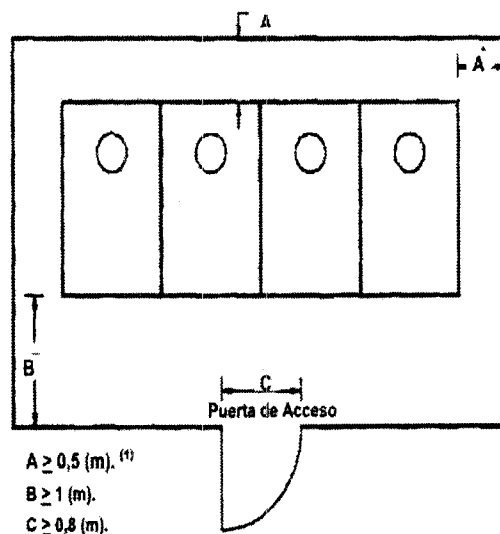
Figura 25. Sala de Calderas - Separadas.
