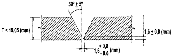
Figura 28. Tubería Exterior - Uniones Soldadas.
