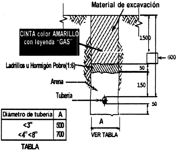
Figura 15. Esquema de Instalación de Tubería Enterrada. - A. Bajo Pavimento
