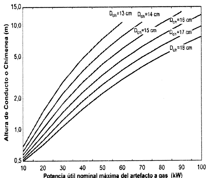
Figura 39. Dimensiones de chimenea para Artefactos de tiro natural a Gas de Ciudad.
