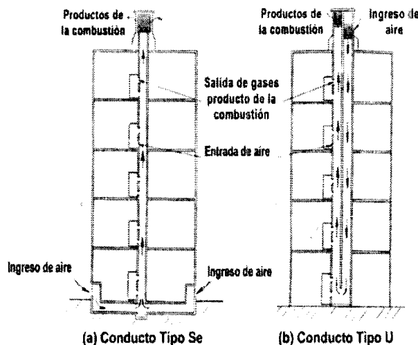
Figura 3. Conductos Colectivos de Evacuación de Gases Producto de la Combustión, Tipos Se y U.
