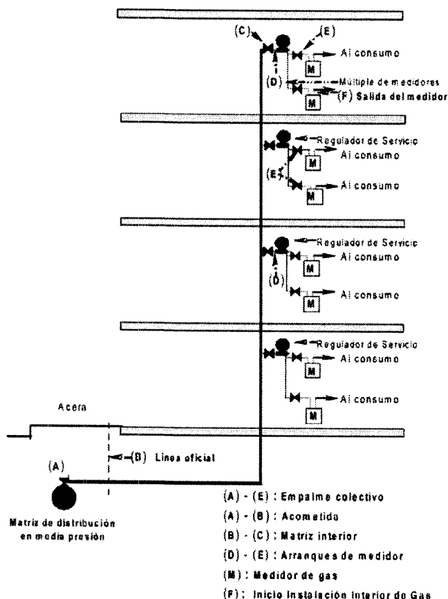
Figura 8. Instalación de Gas – Tipo Condominio.
