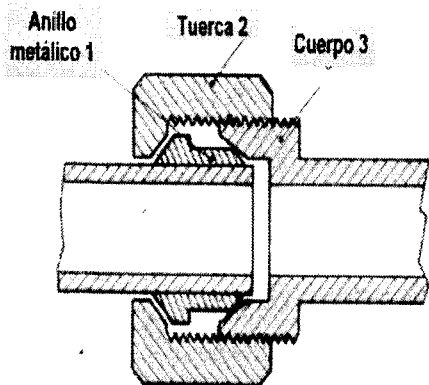
Figura 14. Unión por anillos cortantes.
