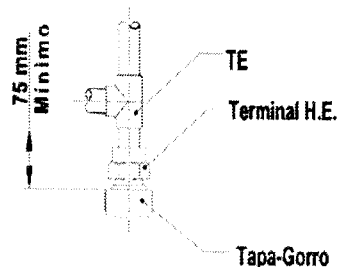
Figura 16. Trampa de sedimentos.
