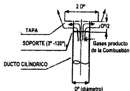
Figura 29. Sombrerete sencillo.
