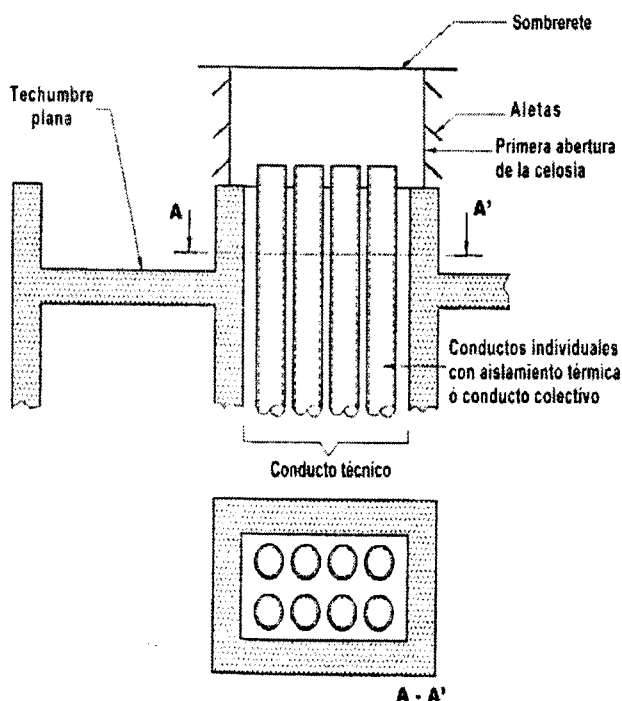
Figura 36. Techumbre Plana con Muros Circundantes – Ubicación del Terminal del Conducto y Sombrerete.
