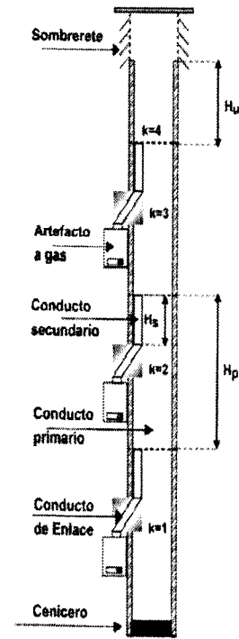
Figura 52. Elementos del Conducto Colectivo de Evacuación de Gases.
