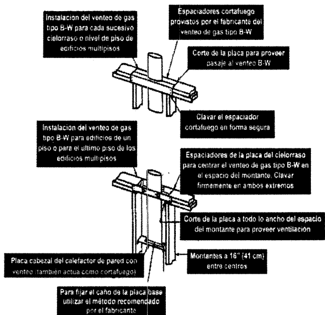
Figura 20. Instalación de un Conducto de Evacuación de Gases del Tipo B-W para Estufas de Pared.
