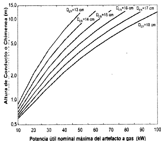
Figura 40. Dimensiones de chimenea para Artefactos de tiro natural a Gas Licuado de Petróleo.
