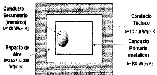
Figura 53. Composición de materiales para el conducto.
