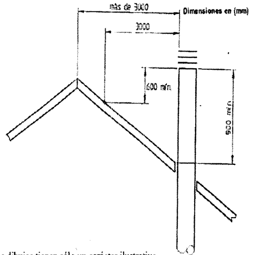
Figura 33. Techumbre – Ubicación del Terminal del Conducto y Sombrerete a más de tres (3) metros del Caballete.
