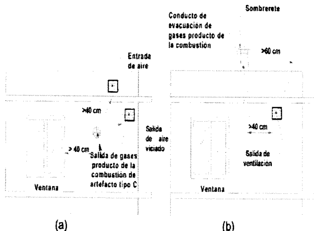
Figura 18. Distancias de las ventilaciones respecto de conductos de evacuación de gases.
