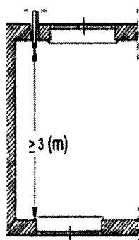
Figura 50. Distancia de Sombrerete a Pared Frontal con Ventana o Ventilación.
