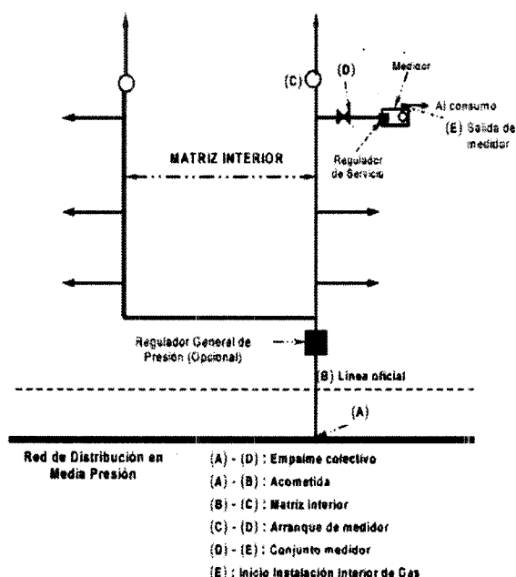
Figura 7. Instalación de Gas con Instalaciones Interiores.
