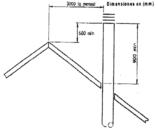
Figura 32. Techumbre – Ubicación del Terminal del Conducto y Sombrerete a tres (3) metros o menos del Caballete.
