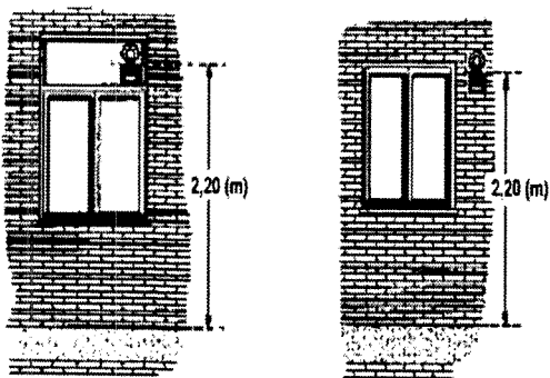
Figura 44. Distancia Mínima de Sombrerete a Ventanas.
