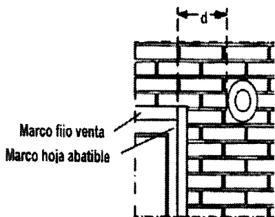
Figura 41. Medición de Distancias.
