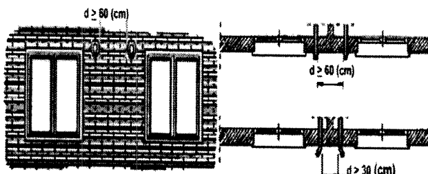
Figura 46. Distancias de Sombreretes al Mismo Nivel.
