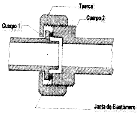
Figura 12. Unión de junta plana o racor.
