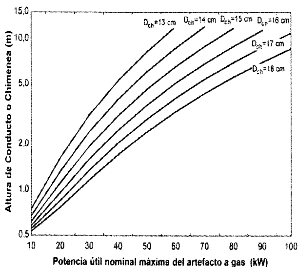
Figura 38. Dimensiones de chimenea para Artefactos de tiro natural a Gas Natural.
