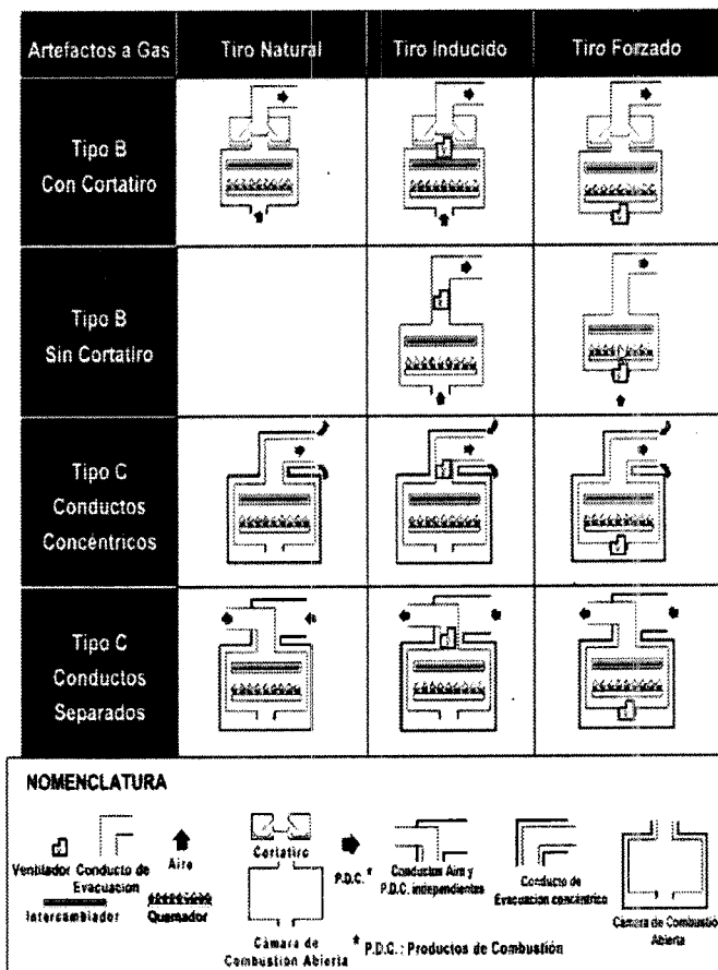
Figura 1. Clasificación de Artefactos a Gas Tipo B y C.
