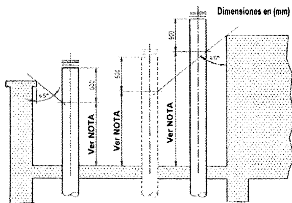
Figura 35. Techumbre – Ubicación del Terminal del Conducto y Sombrerete a más de tres (3) metros de un Muro o Antepecho.
