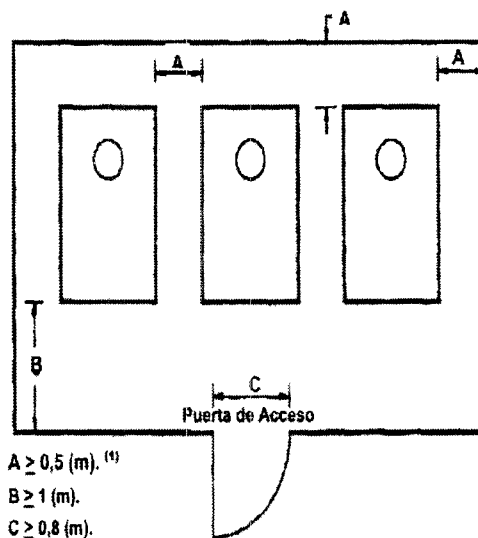
Figura 24. Sala de Calderas - Quemador Acoplado.
