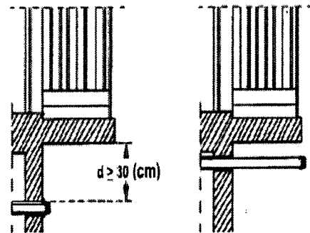
Figura 47. Distancia de Sombrerete bajo Balcón.
