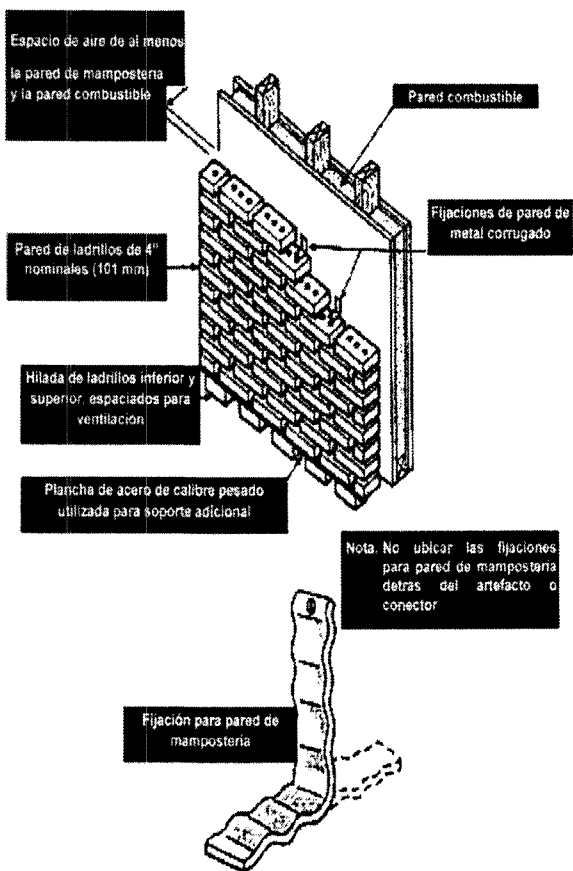
Figura 23. Sistema de Reducción del Espacio Libre de Mampostería.
