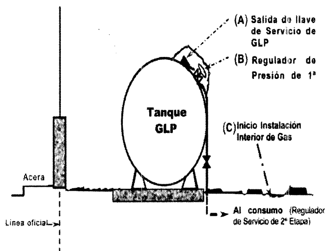
Figura 5. INSTALACIÓN INTERIOR DE GAS CON EQUIPO DE GLP.
