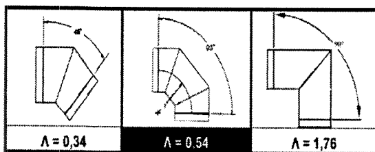
Figura 54. Coeficientes de pérdidas de carga para codos.
