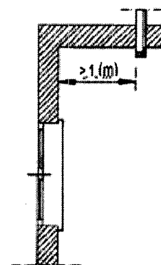
Figura 48. Distancia de Sombrerete a Pared Lateral con Ventana o Ventilación.
