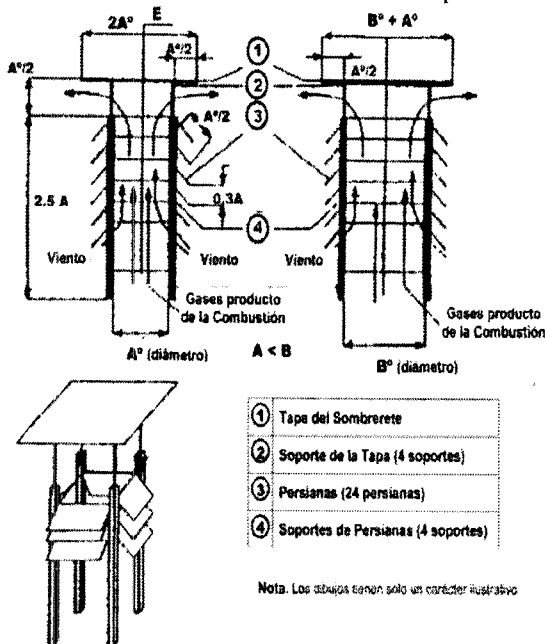
Figura 31. Sombrerete aspirador estacionario.
