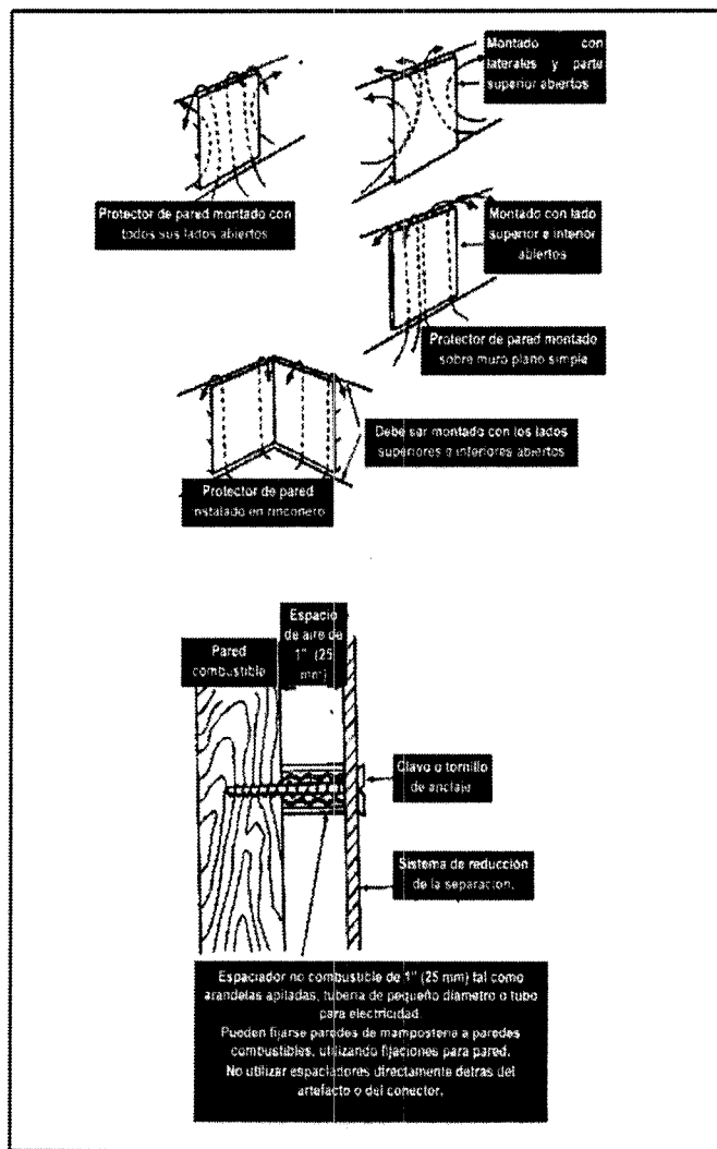
Figura 22. Sistema de Reducción del Espacio Libre con Protector de Pared.
