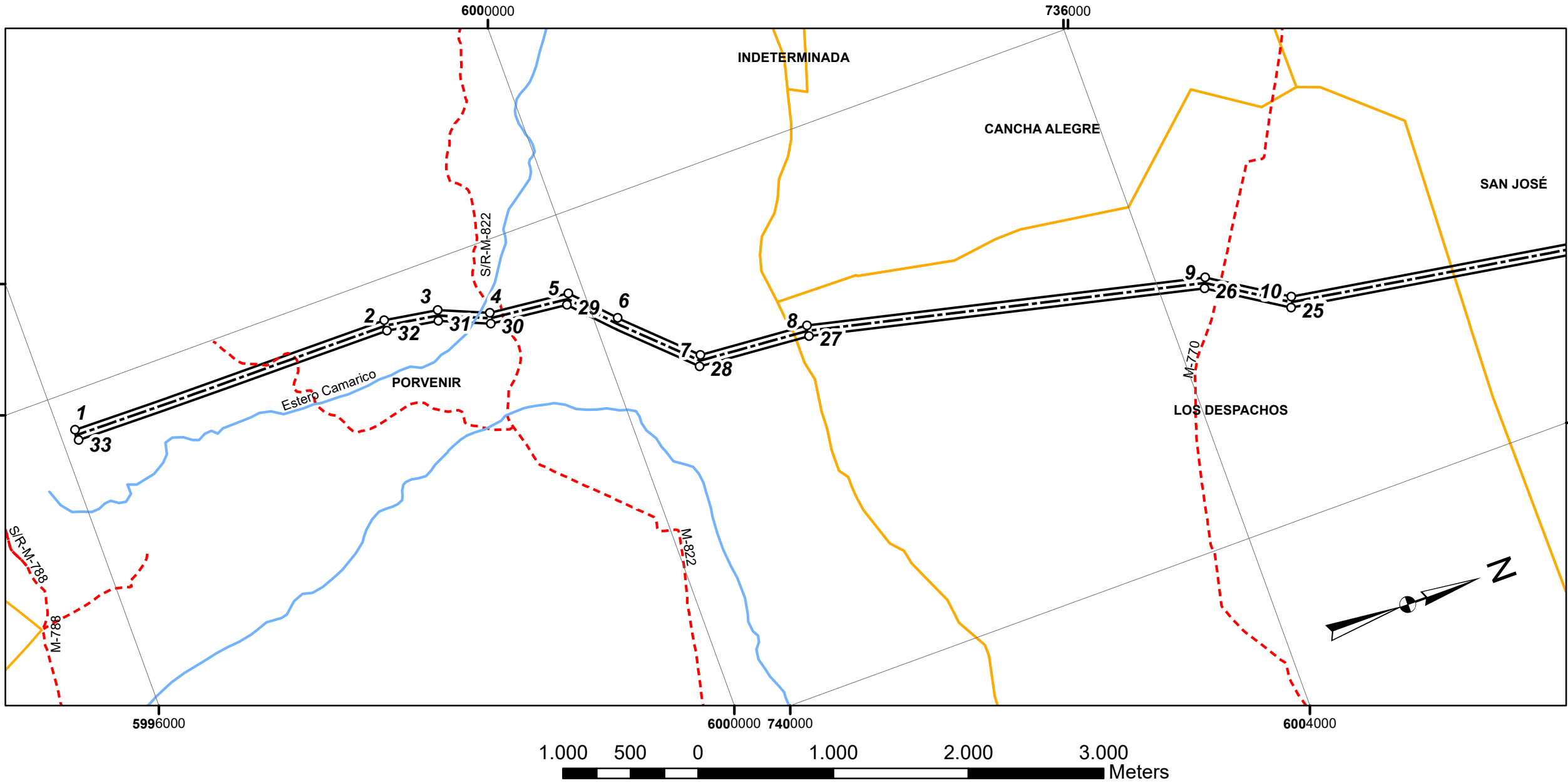
PLANTA DETALLE 3
