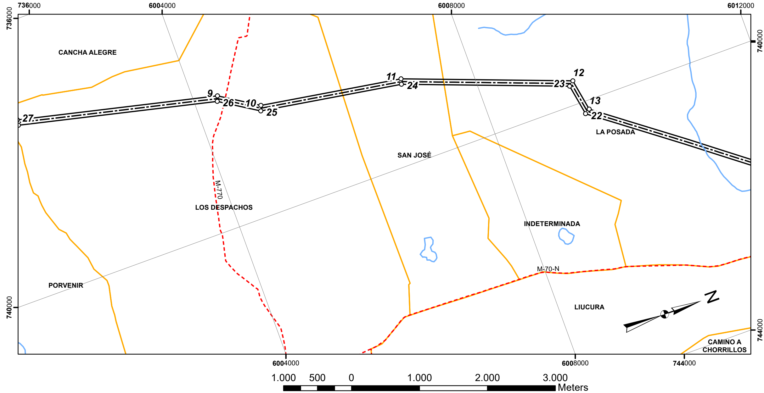
PLANTA DETALLE 2
