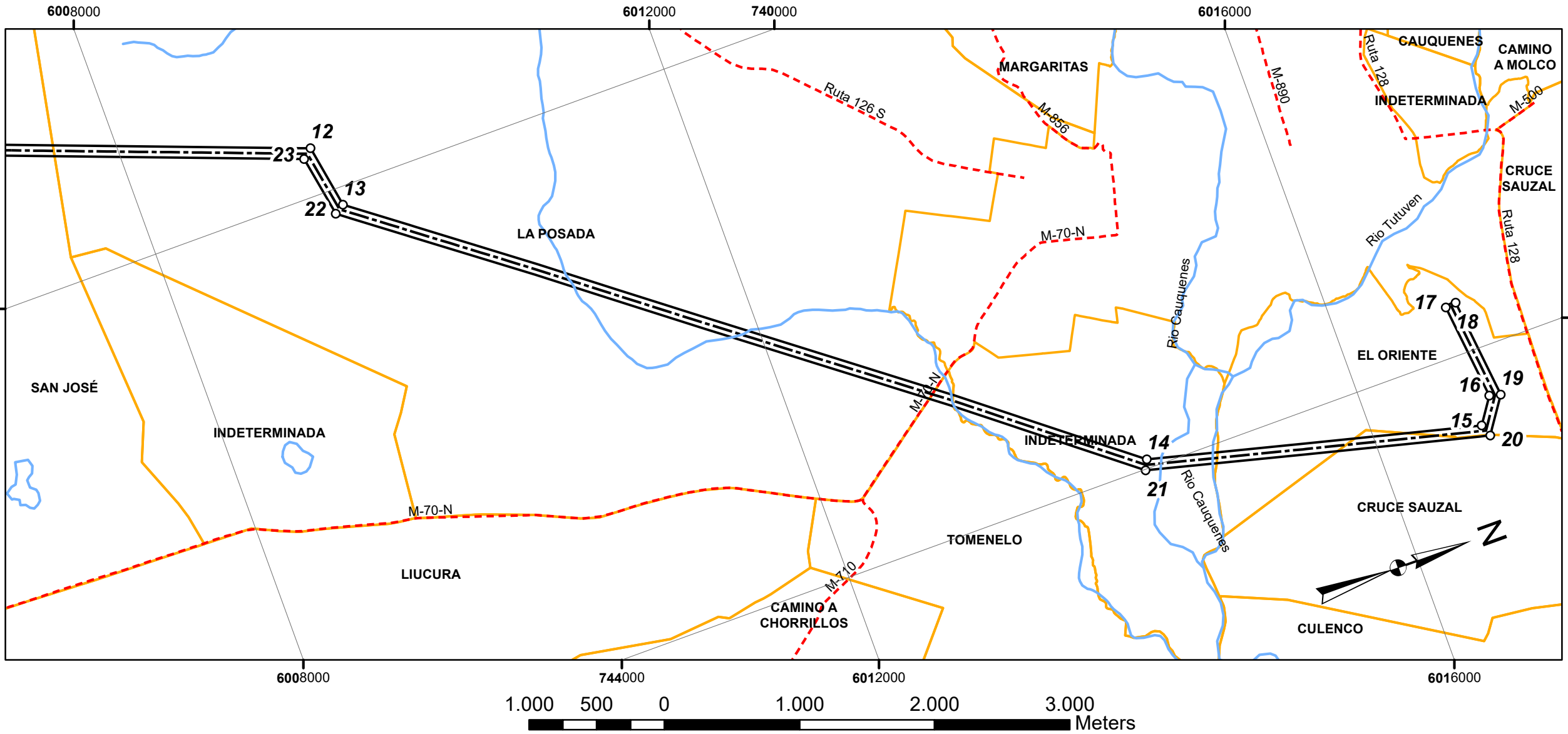
PLANTA DETALLE 3
