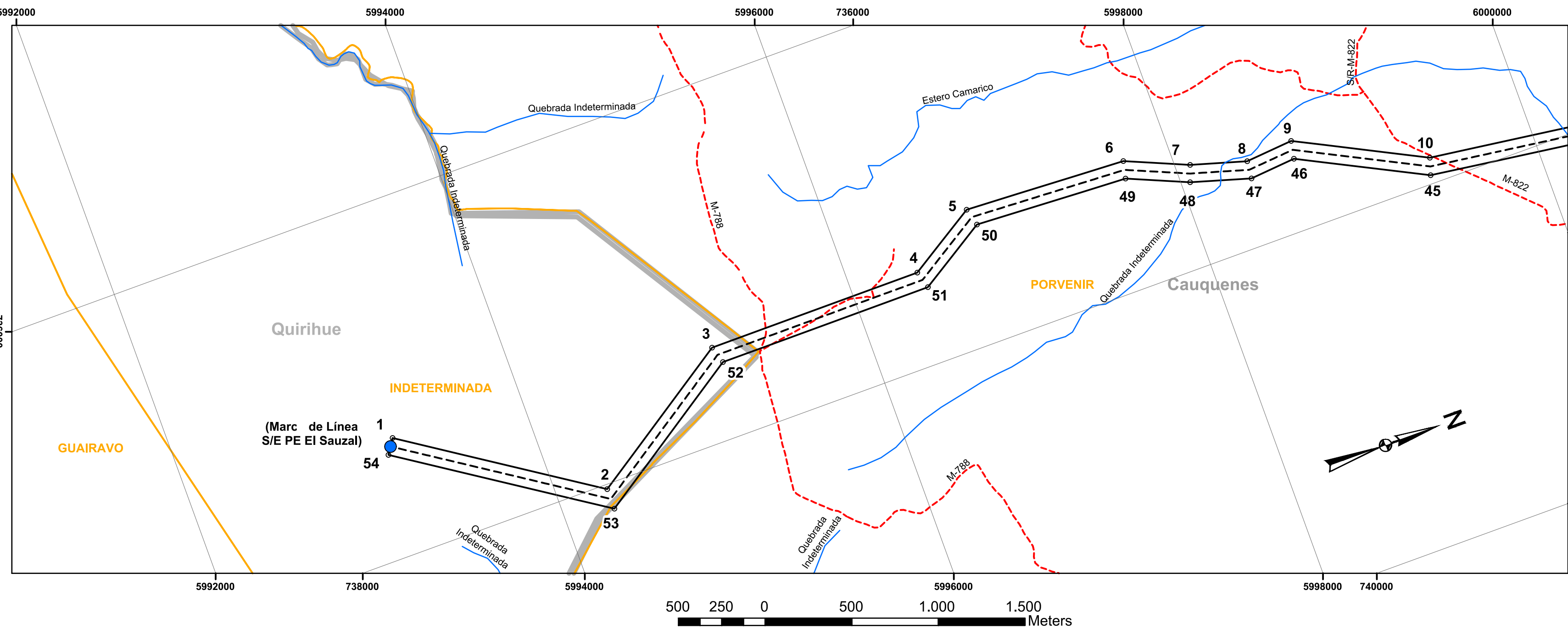
PLANTA DETALLE 3
