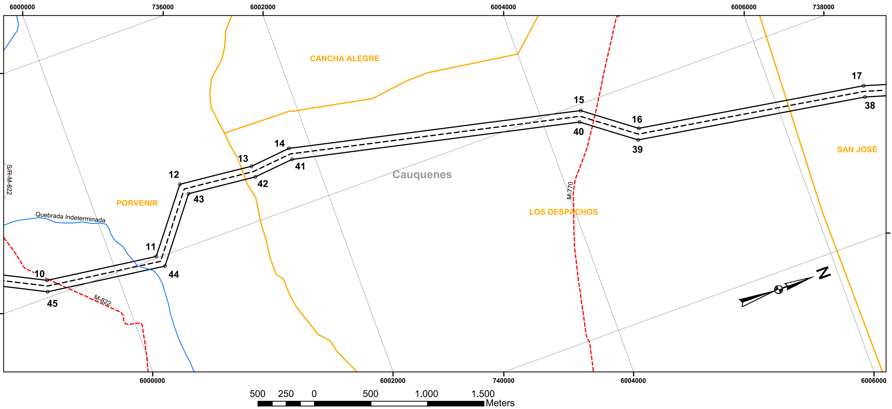
PLANTA DETALLE 2
