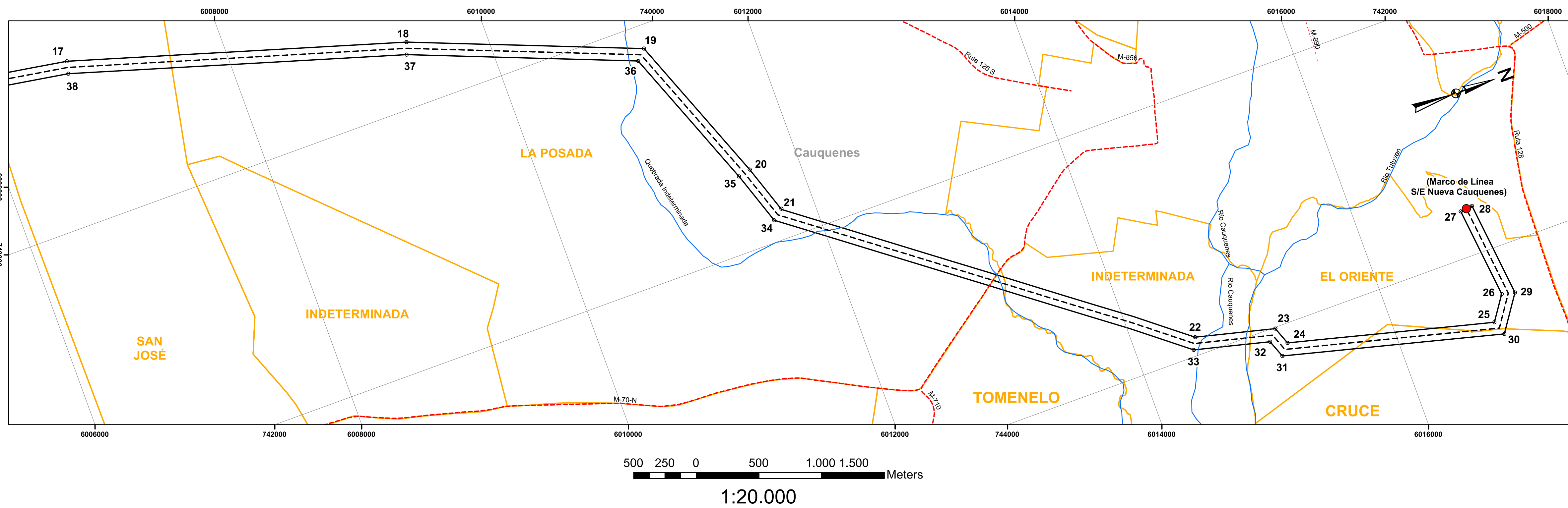
PLANTA DETALLE 3
