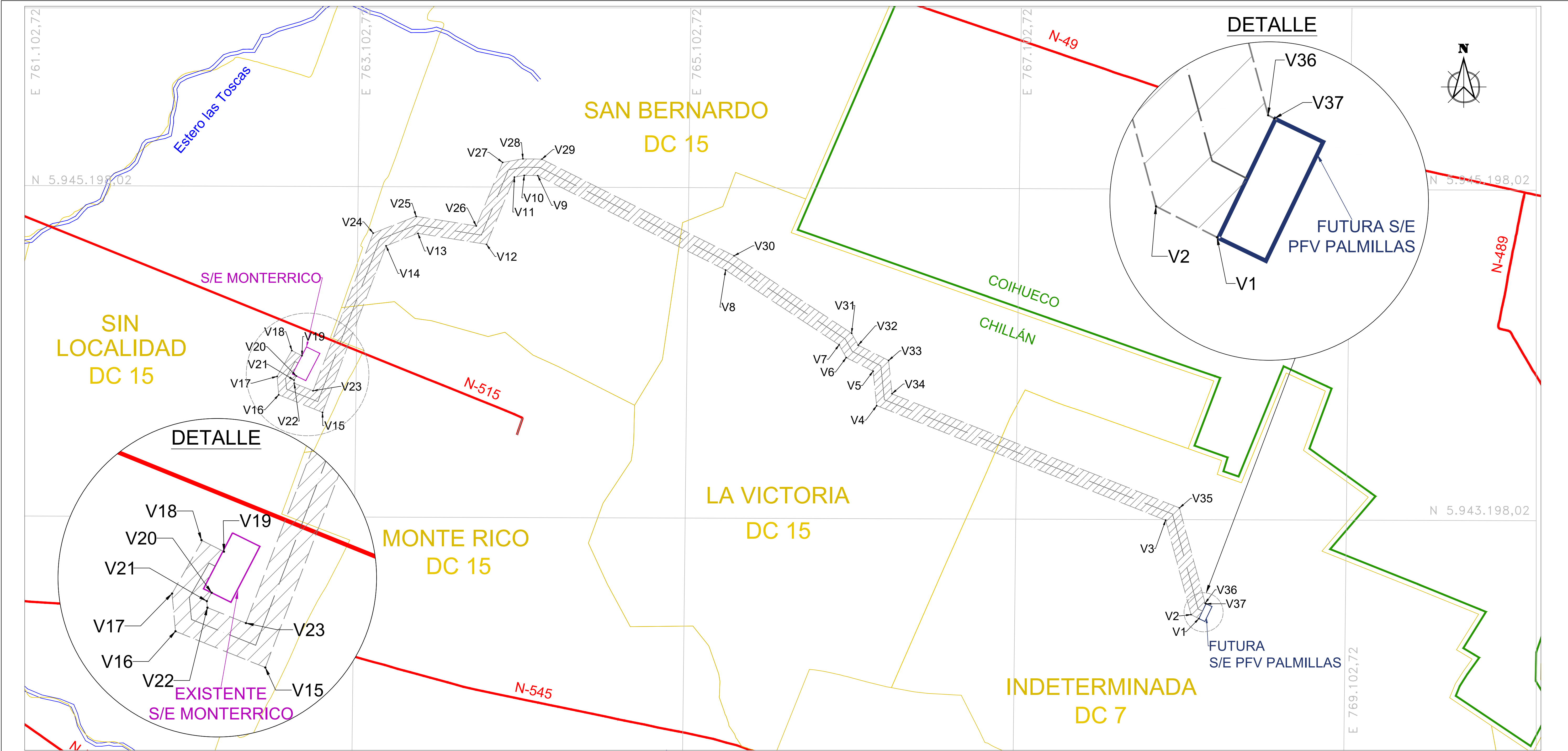
DETALLE EN PLANTA: LÍNEA DE TRANSMISIÓN 1x220kV PFV PALMILLAS – S/E MONTERRICO
